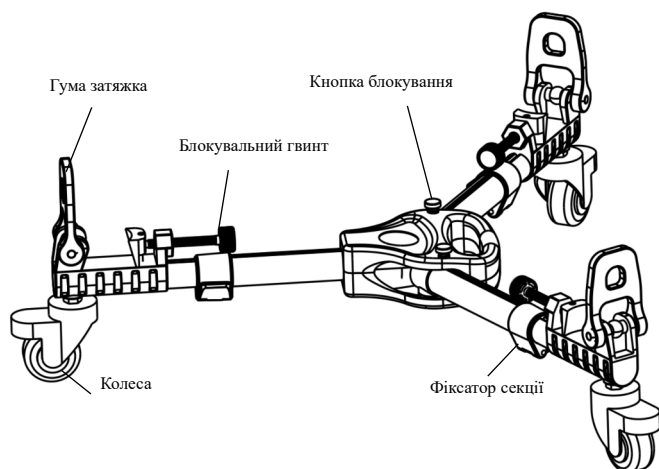
Штативний візок
